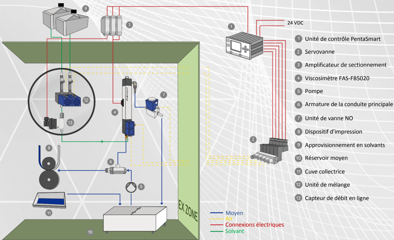
(Fig. S6-FB Système de mesure de la viscosité avec option de mélange pour 2 solvants)
