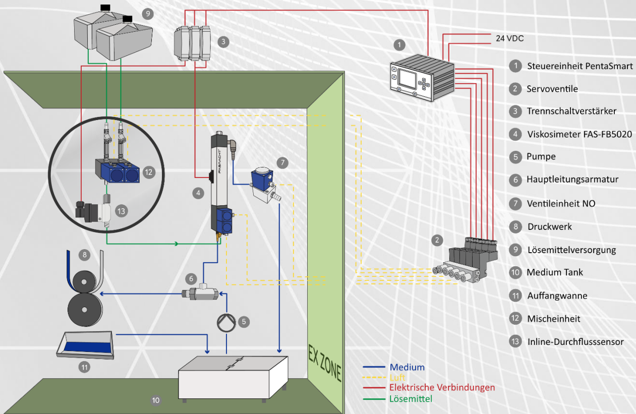
(Abb. S6-FB Viskositätsregelsystem mit Option Mischen für 2 Lösemittel)
